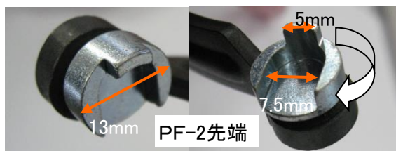
PF-1先端 内径φ 8mm 外径φ 13mm
