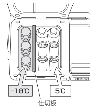
仕切板
