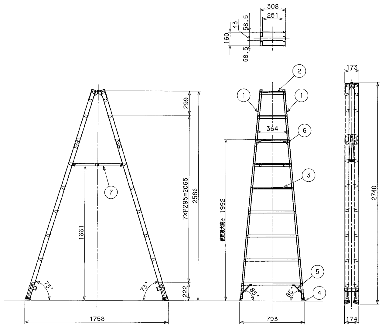
収納状態
