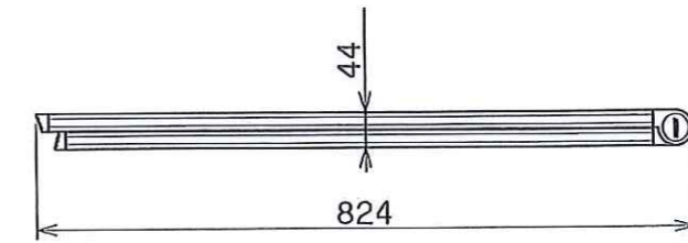
収納寸法
