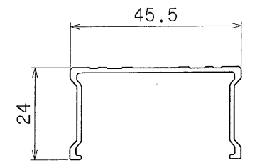
支柱断面図 (1/1)
