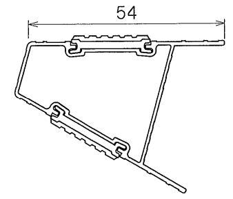
踏棧断面図 (1/1)
