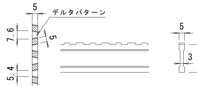
DI-25 バー形状詳細 S=1:2
