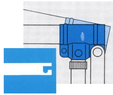
ポンプ部は狭い場所でも動かせるようデザインされています。ジャッキを車の下に押し込んだ後でハンドルを差し込む事ができます。
