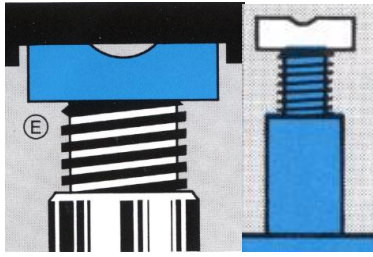
サドルは丸型でネジによる調整可能
